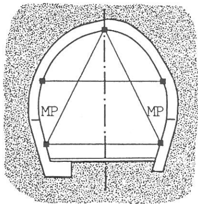
Fig. 5 Sezione equipaggiata con chiodi per le misure di convergenza, e con martinetti piatti (MP) per il controllo della tensione circonferenziale nel rivestimento.
