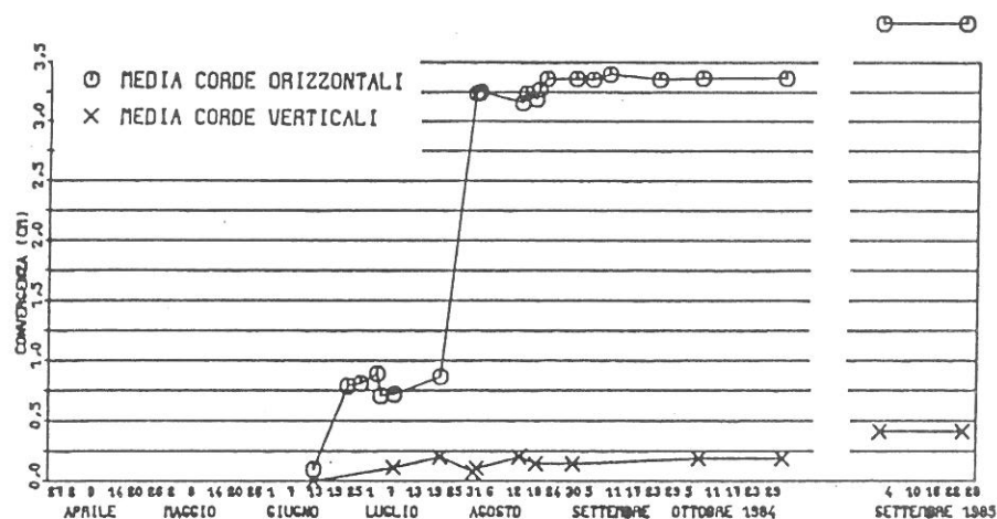
Fig. 6 Sezione C1 - Misure di convergenza: la chiusura della sezione è in gran parte dovuta agli effetti delle iniezioni eseguite a fine luglio.
